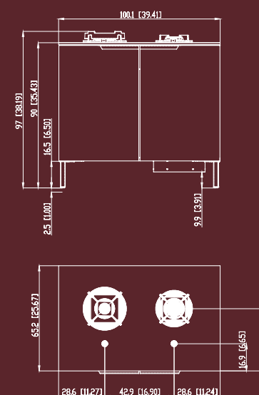
Burner Module 100
