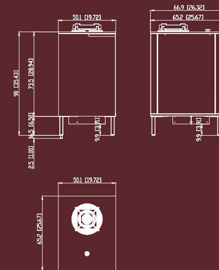
Burner Module 50
